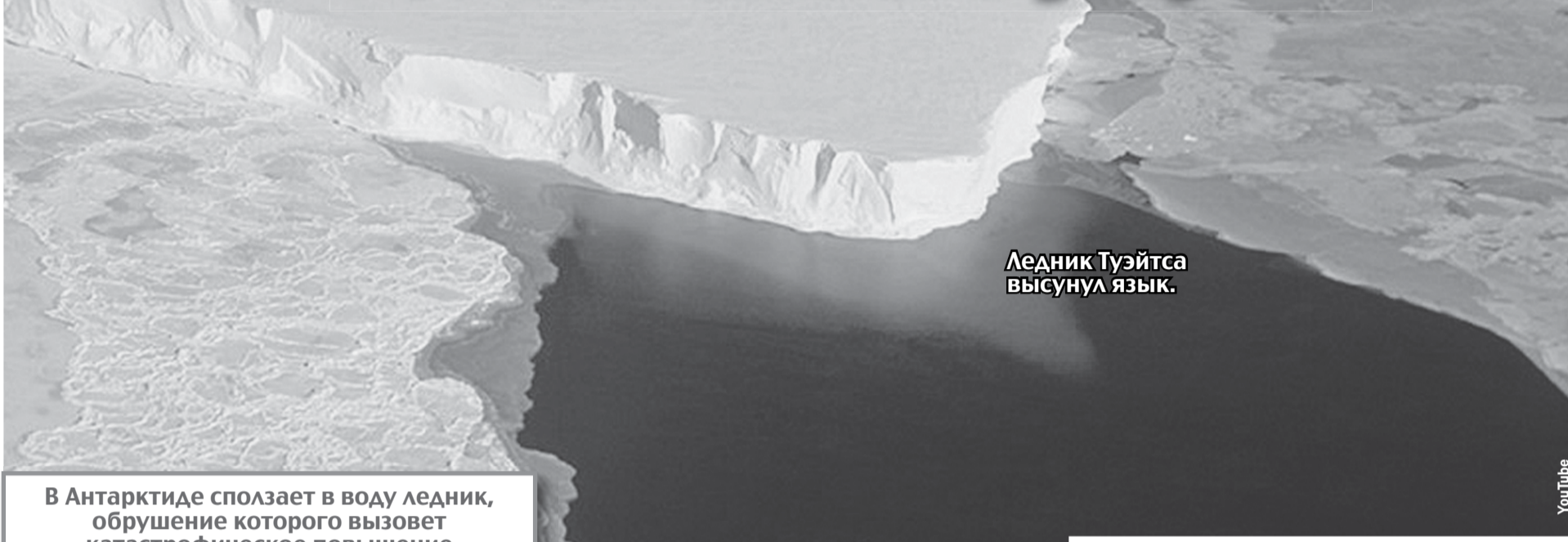
ЛЕДНИК ТУЭЙТСА
